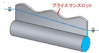
◆ 満管の流れ(管水路モデル)
