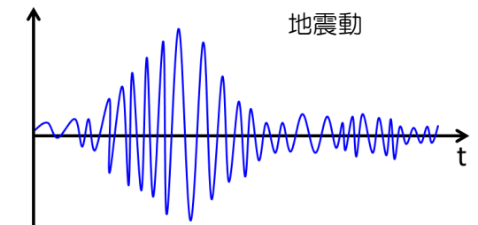
地震動による地盤の液状化と沈下
