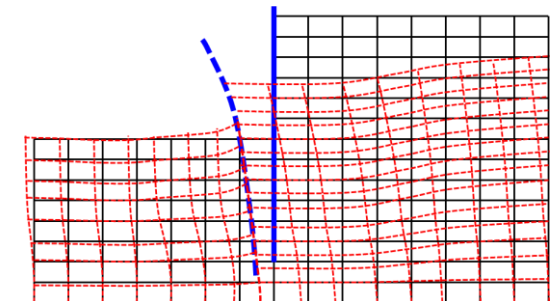
液状化による沈下・側方流動
